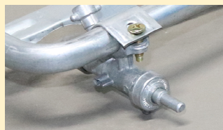
Válvula de Segurança sem “Castelo” (Antiga)
